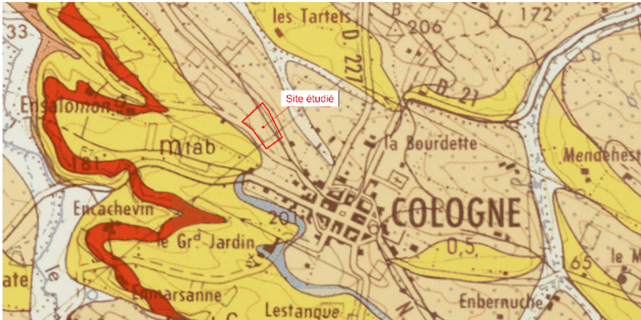
Figure 2 – Contexte géologique – Source : Géoportail
