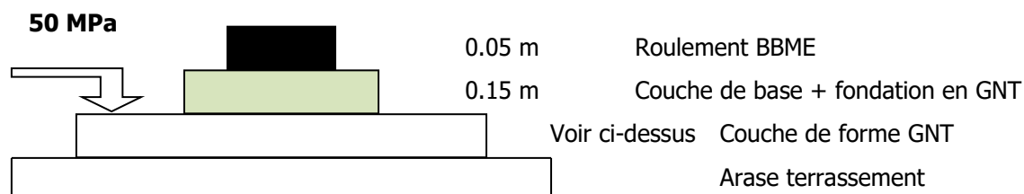
Schéma de la structure de voirie
